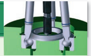
内側から爪を引掛け、溝付きベアリングを傷つけずに引き抜きます
